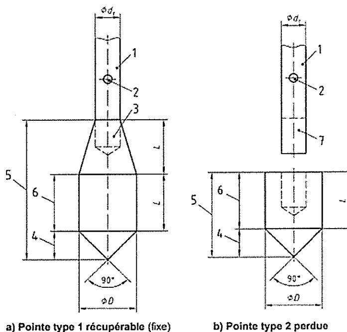
Figure 1 — Formes alternatives de pointe pour essais de pénétration dynamique
